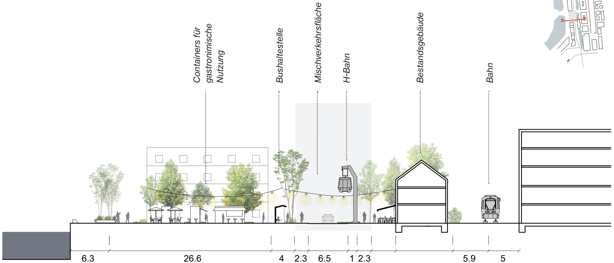
Schnitt A-A' Die Verschwenkung des Straßenverlaufs am Siloplatz schafft einen Aufenthaltsbereich vor dem Bestandsgebäude
