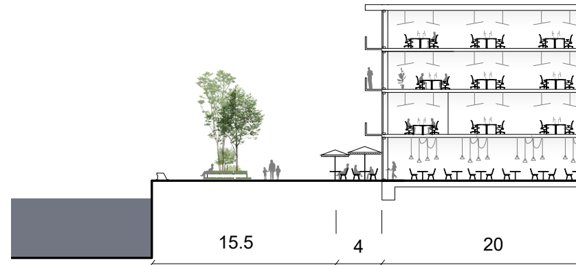
Hafenpromenade Schnitt
